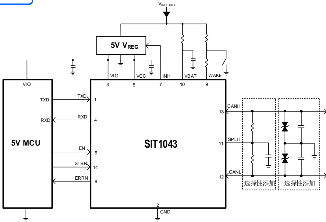
图 10 SIT1043 与 5V MCU 的典型应用图
