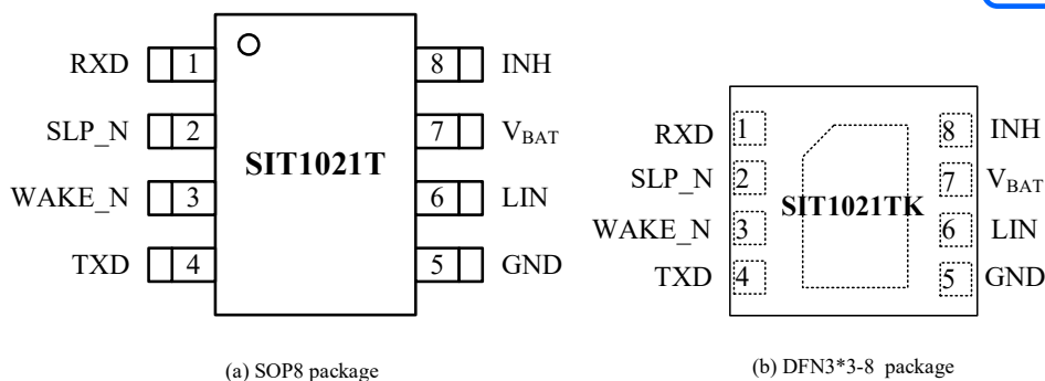
图 2 SIT1021 引脚分布图
