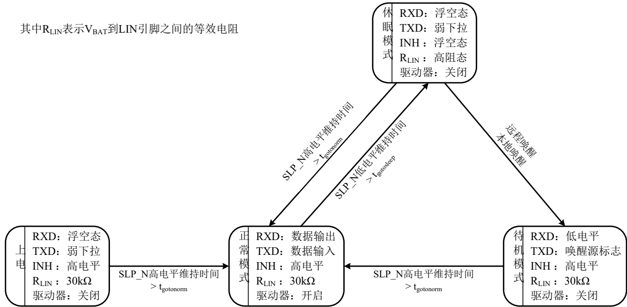
图 4 状态转换图
