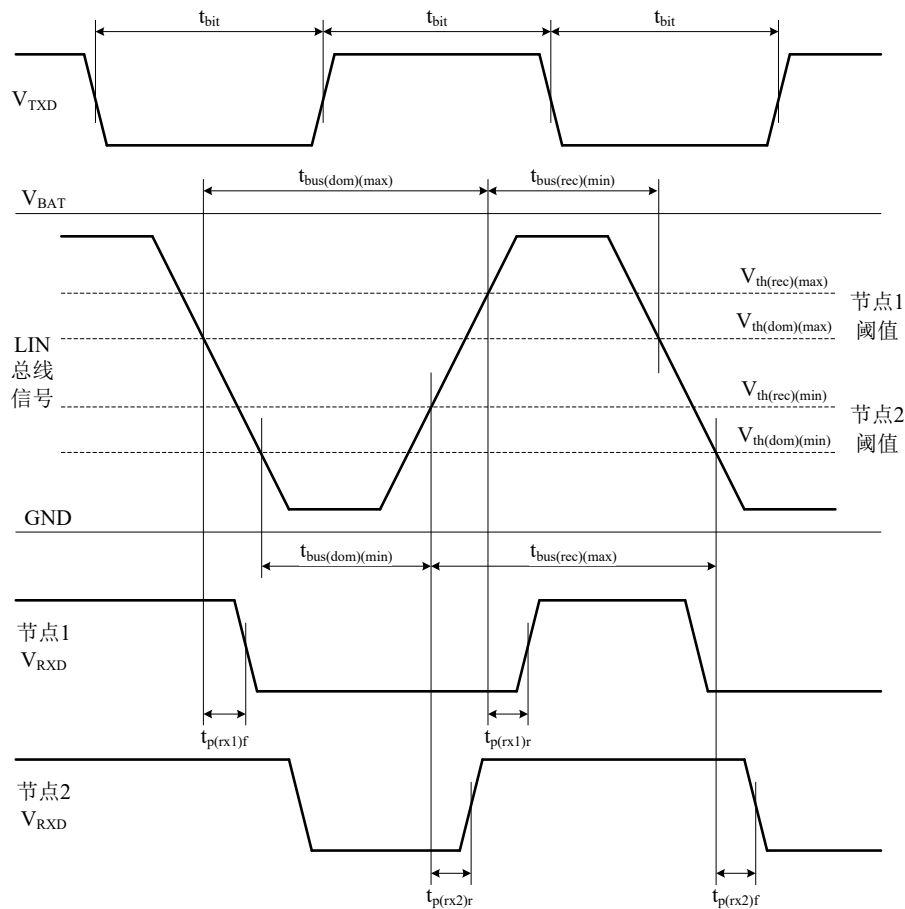
图 6 总线信号传输时序图
