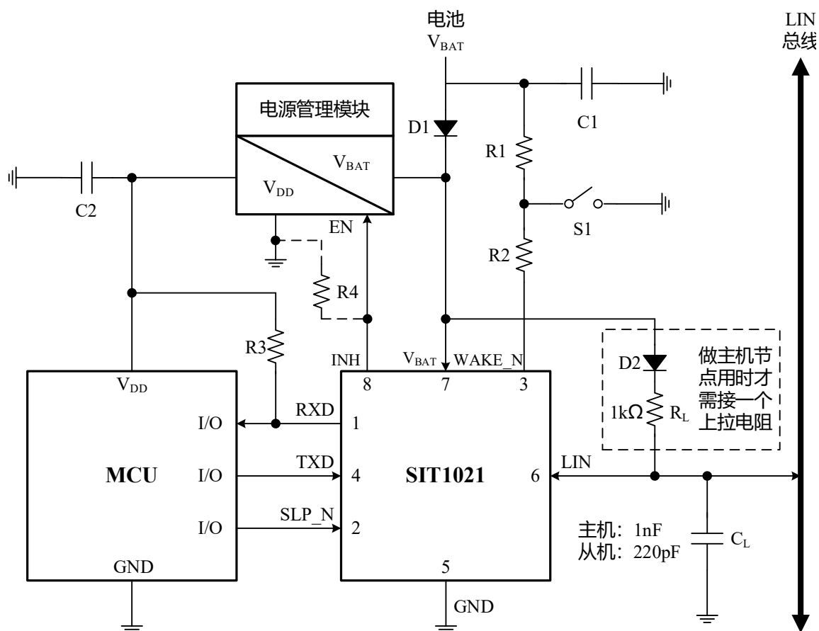
图 7 SIT1021 典型应用示意图
