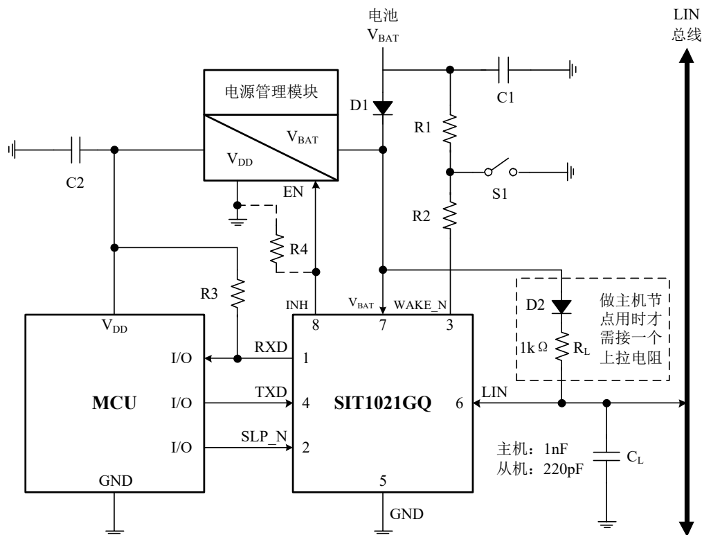
图 6 SIT1021GQ 典型应用示意图
