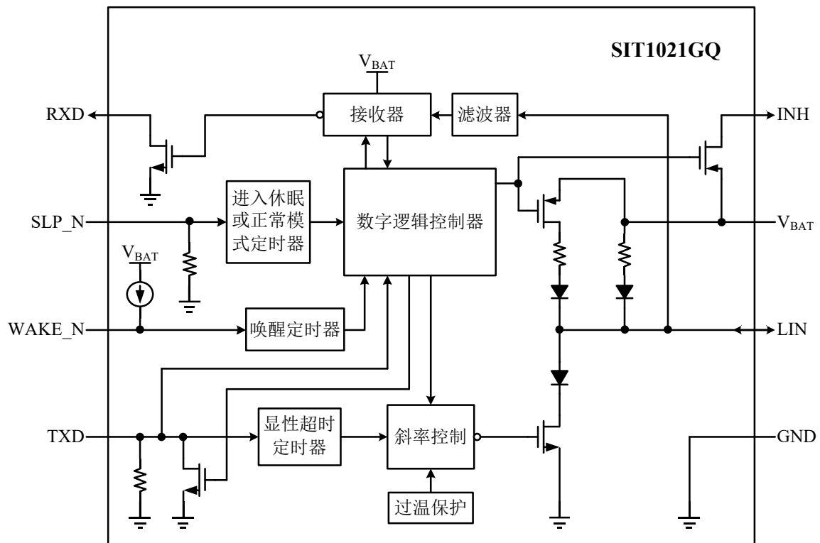
图 2 SIT1021GQ 内部框图
