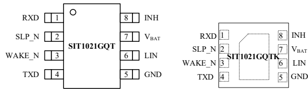
图 1 SIT1021GQ 引脚分布图
